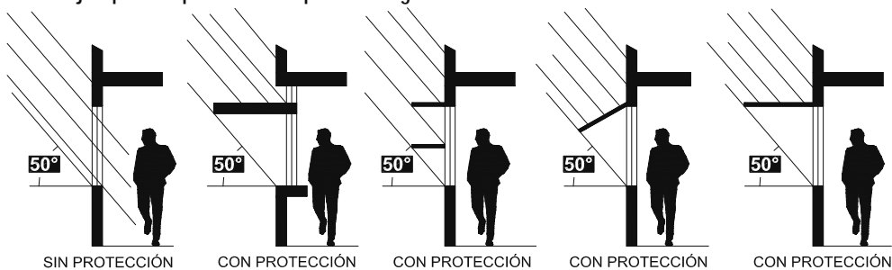
Ejemplos de protecciones para un ángulo de 50°
