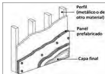
Ejemplo de sistema constructivo en seco con perfiles metálicos que sobresalen del panel prefabricado
